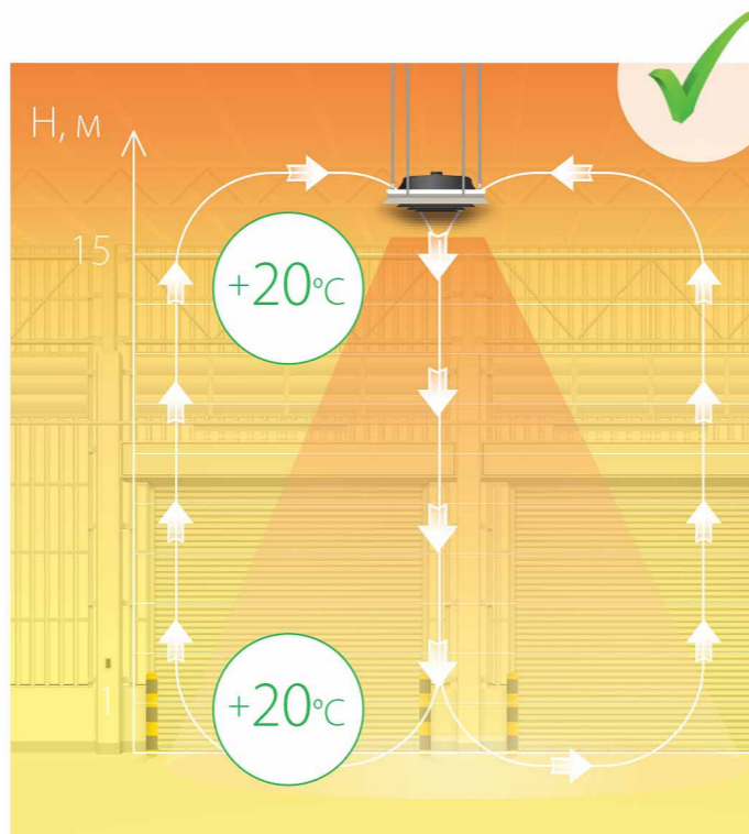
Распределение тепла в здании с использованием дестратификаторов
